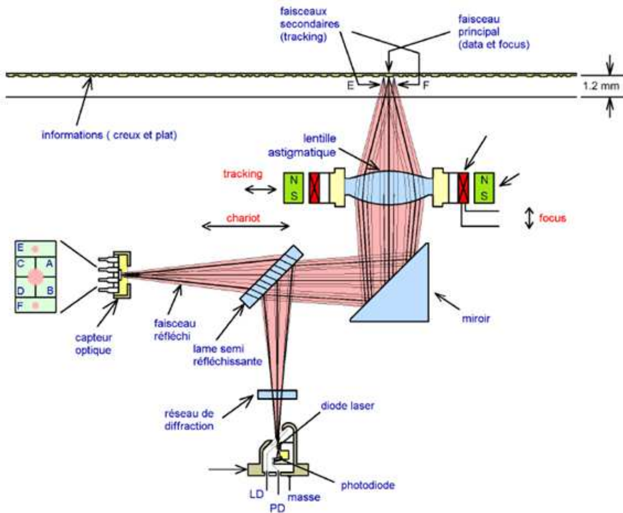
Le système optique à 3 faisceaux
